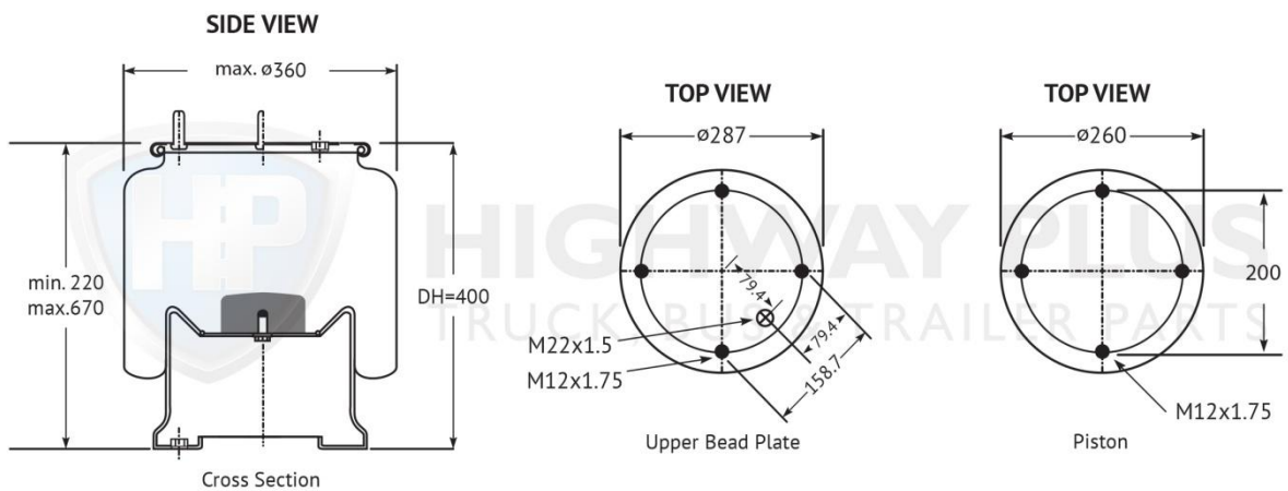
HP301-119 Airbag York Tecair 1
