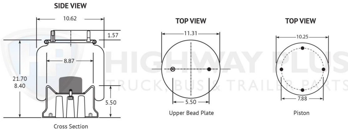
HP301-114 Airbag York Tecair FB3 Duratrac
