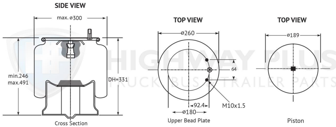
HP301-128 Airbag Volvo Scania
