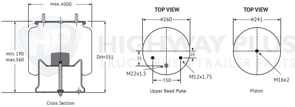
HP301-123 Airbag SAF 2619V SAF Intradisc
