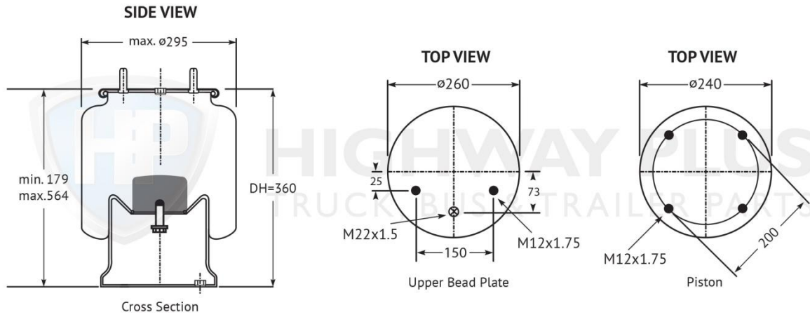
HP301-122 Airbag SAF 2618V
