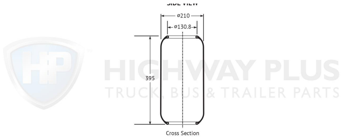
HP301-126 Airbag Volvo, Mercedes
