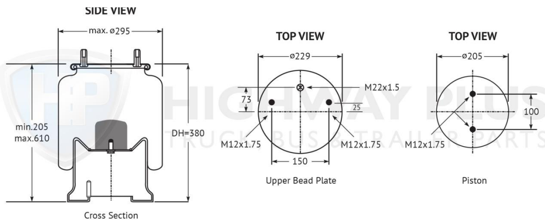
HP301-103 Airbag Holland E510 E520 E530 U514 ROR
