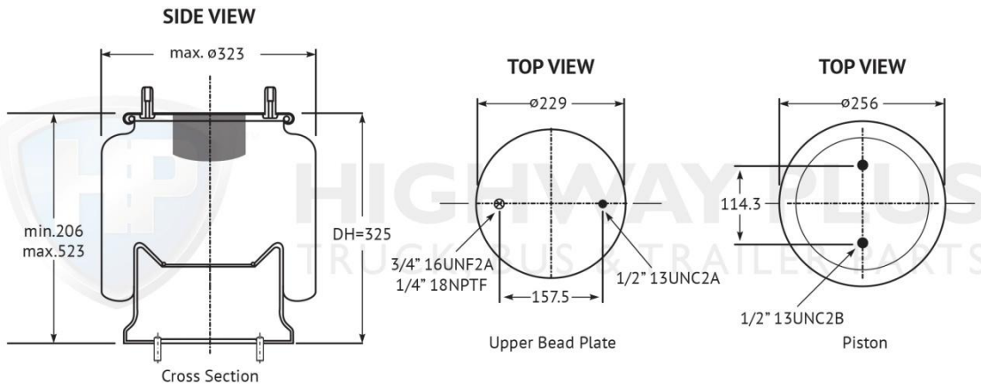
HP301-109 Airbag Hendrickson HA & WD
