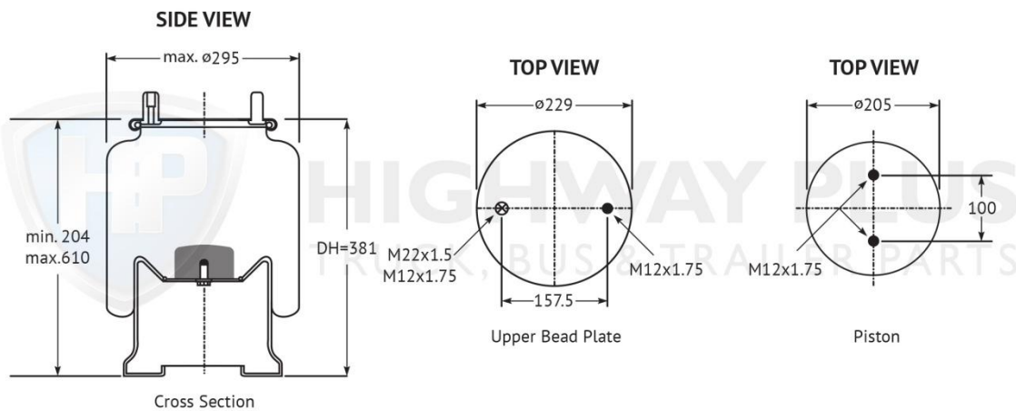
HP301-102 Airbag ROR-Meritor
