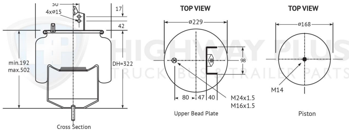
HP301-129 Airbag Volvo FM9
