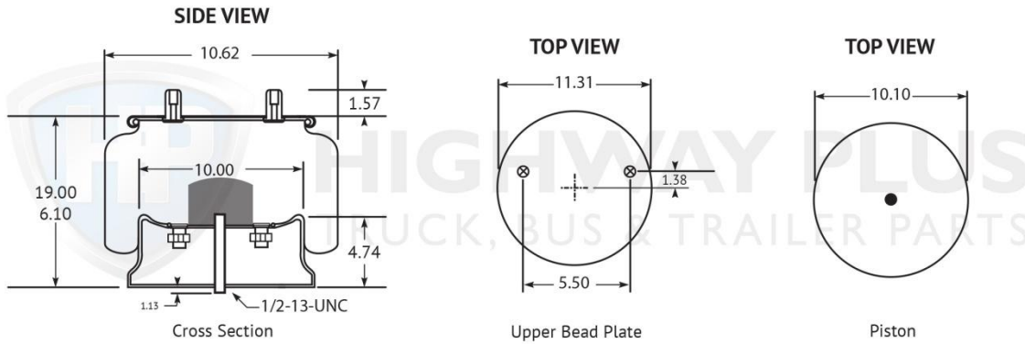
HP301-118 Airbag Hendrickson Intraax AA250
