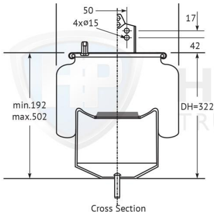
HP301-132 Airbag Volvo
